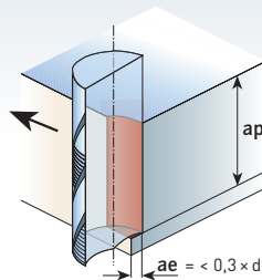
Umfangfräsen/Schichten Circumference milling/Finishing
